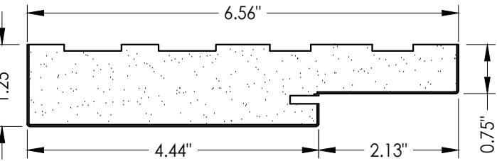
1 POLY FIBER JAMB
